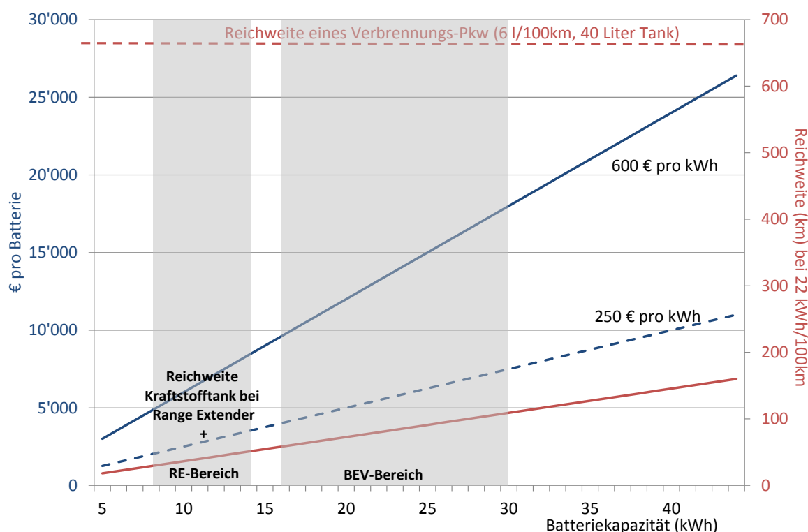
Abbildung 68: Batteriekosten und Fahrzeugreichweite nach Batteriekapazität
