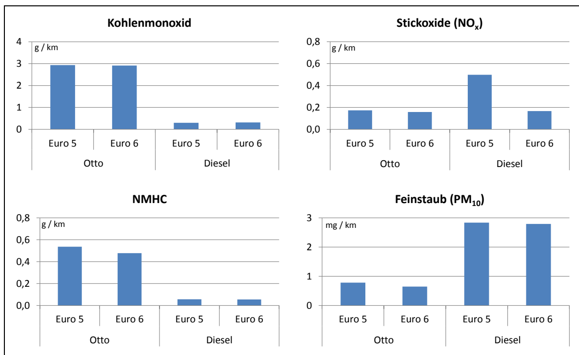
Abbildung 24: Emissionsfaktoren (Innerorts) ausgewählter Schadstoffe nach HBEFA
