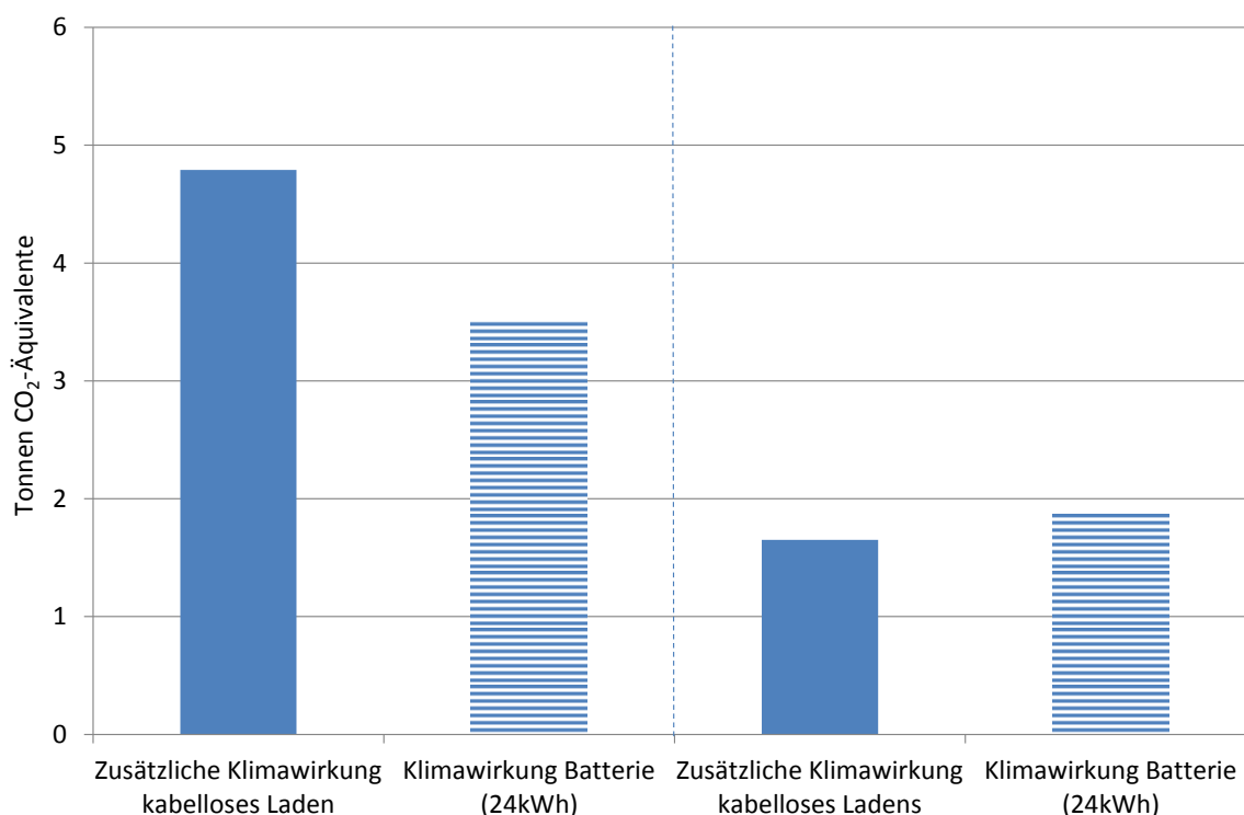
Abbildung 66: Zusätzliche Treibhausgasemissionen induktives Laden im Vergleich zur Batterieherstellung
