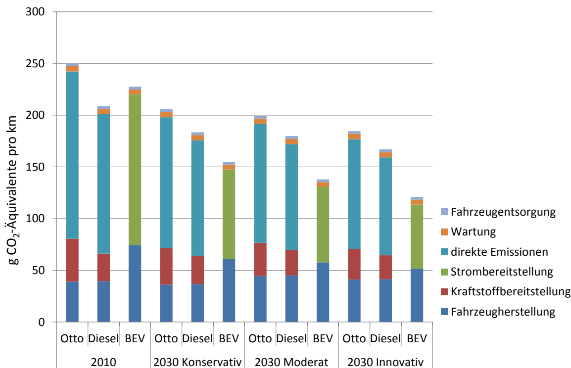
Abbildung 61: Treibhausgasemissionen eines mittleren Otto-, Diesel- und BEV-Pkw in Szenarien (2030)
