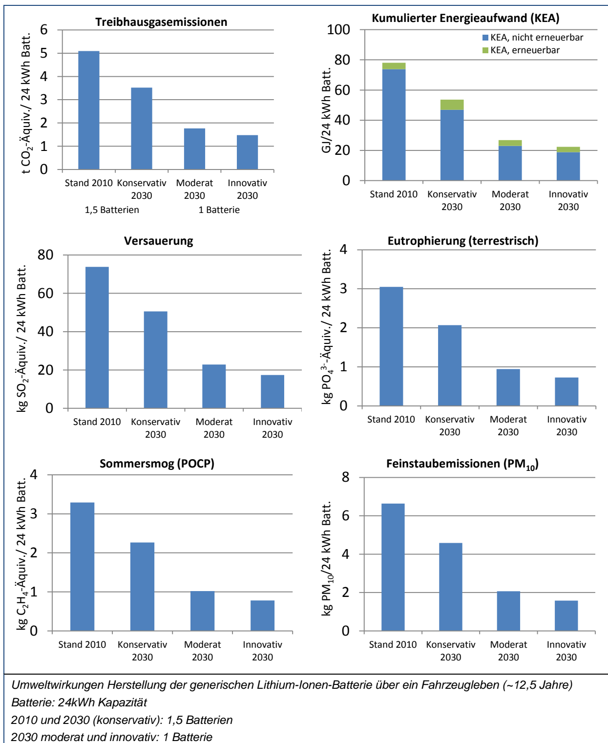
Abbildung 11: Umweltbilanzen für die Batterieherstellung
